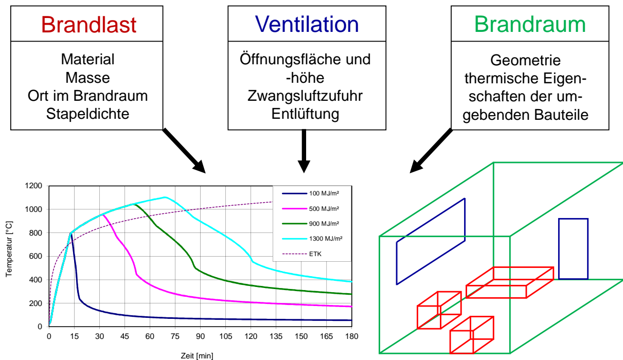
Bild 2 Einflussparameter eines Brandes und zeitlicher Verlauf der Heißgastemperatur bei unterschiedlichen Brandlastdichten
